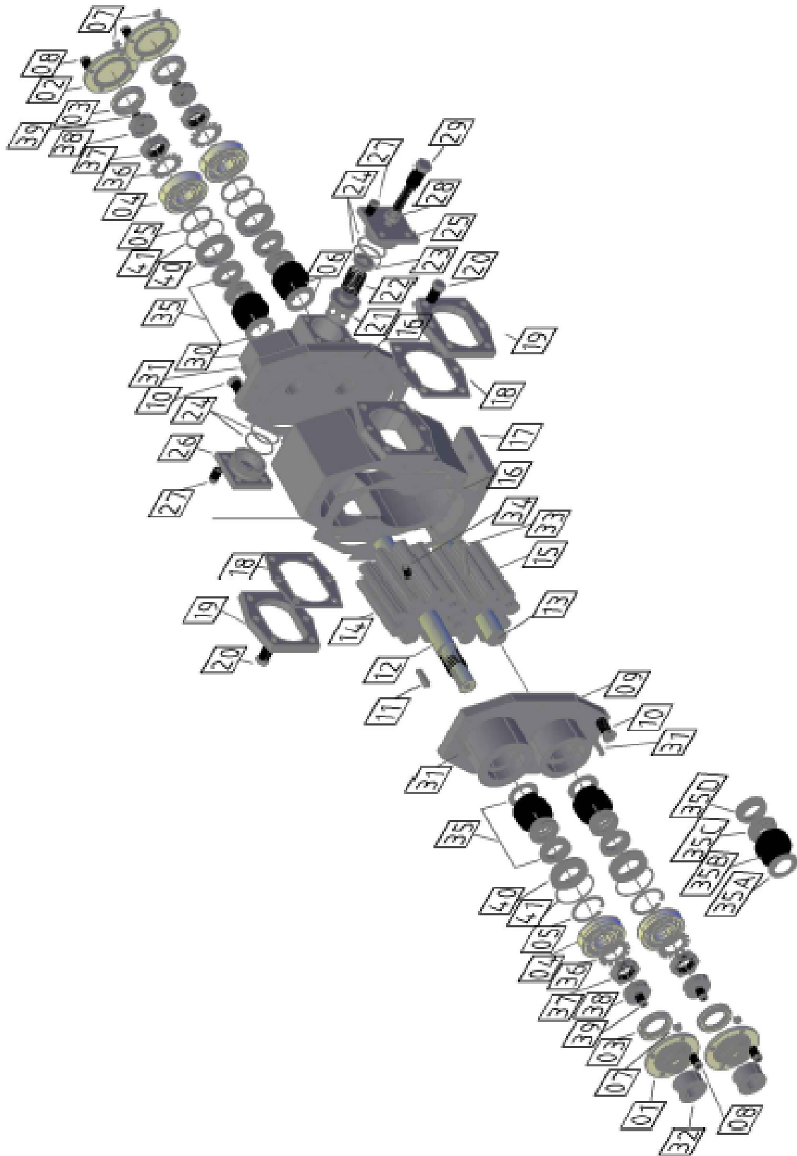
Εικόνα 7: Ανταλλακτικά αντλίας 4''
