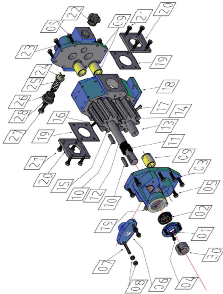
Εικόνα 5: Ανταλλακτικά αντλίας 1 1/2"
