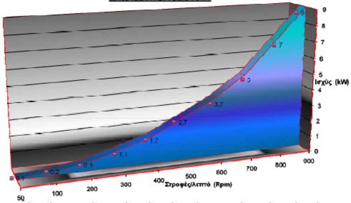
Διάγραμμα Ισχύος-Στροφών
