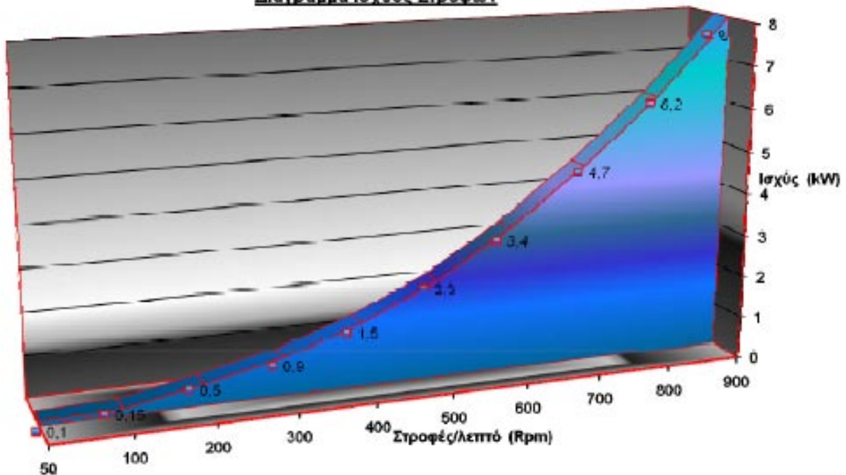
Διάγραμμα Ισχύος-Στροφών
