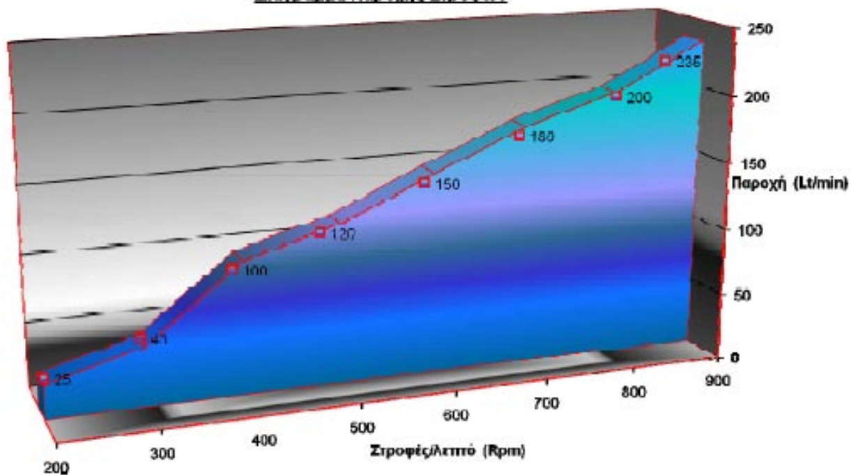
Διάγραμμα Παροχής-Στροφών
