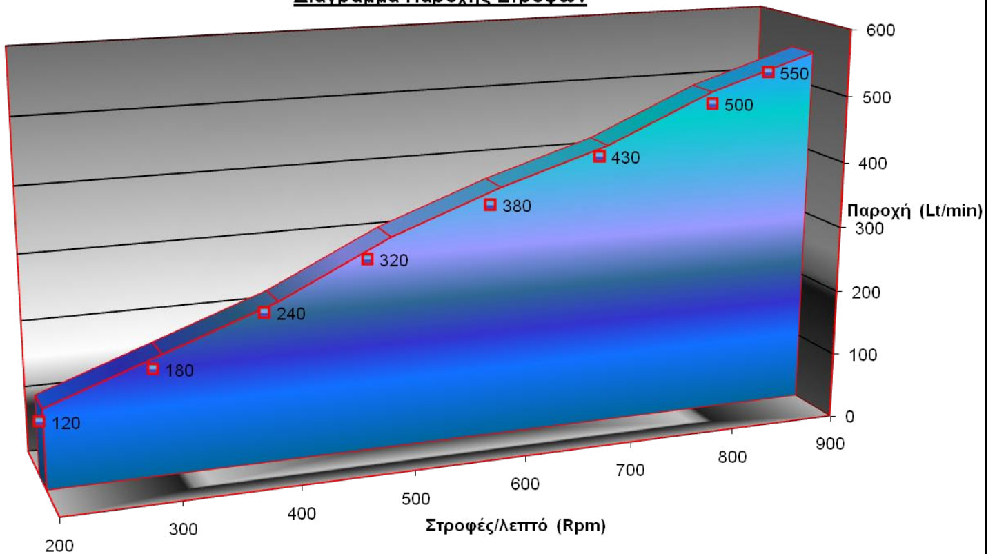
Διάγραμμα Παροχής-Στροφών
