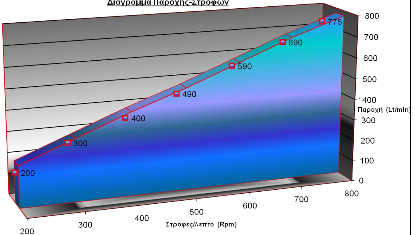
Διάγραμμα Παροχής-Στροφών
