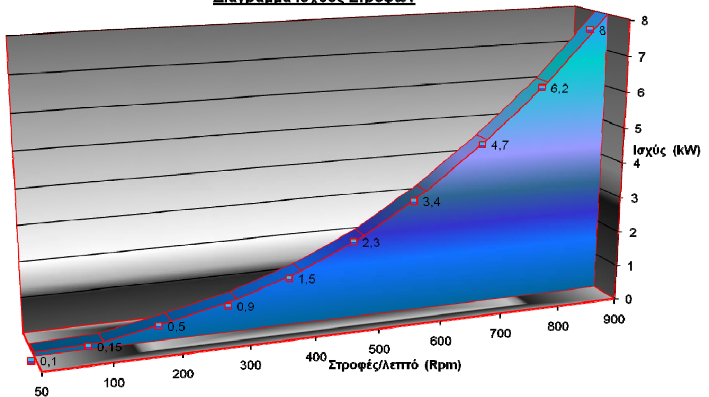
Διάγραμμα Ισχύος-Στροφών
