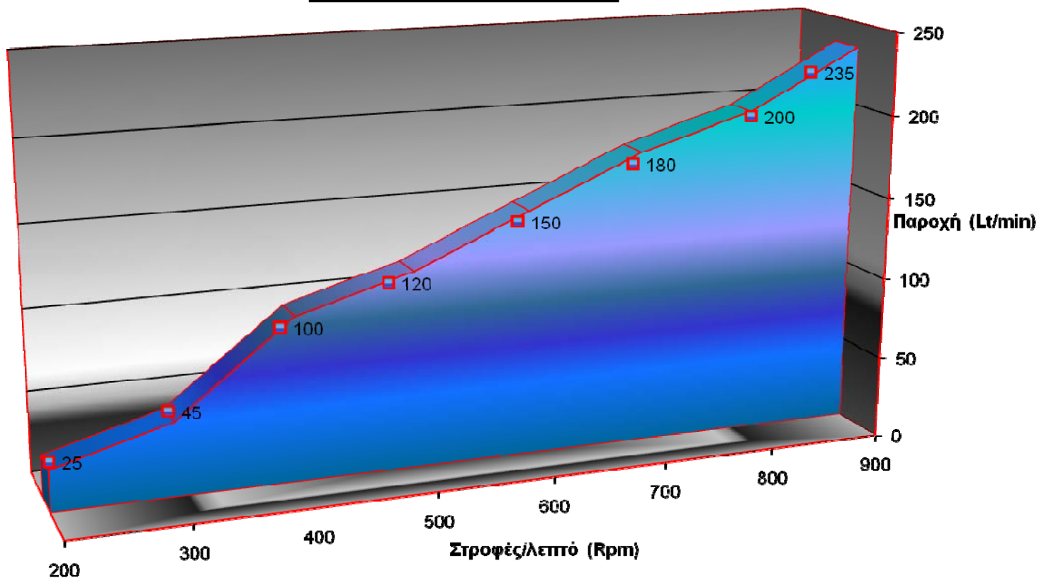
Διάγραμμα Παροχής-Στροφών
