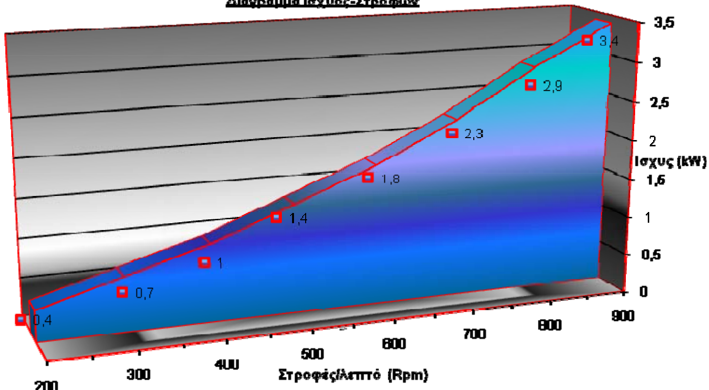
Διάγραμμα Ισχύος-Στροφών
