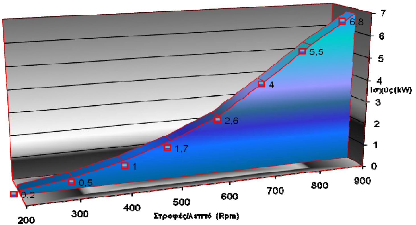
Διάγραμμα Ισχύος-Στροφών
