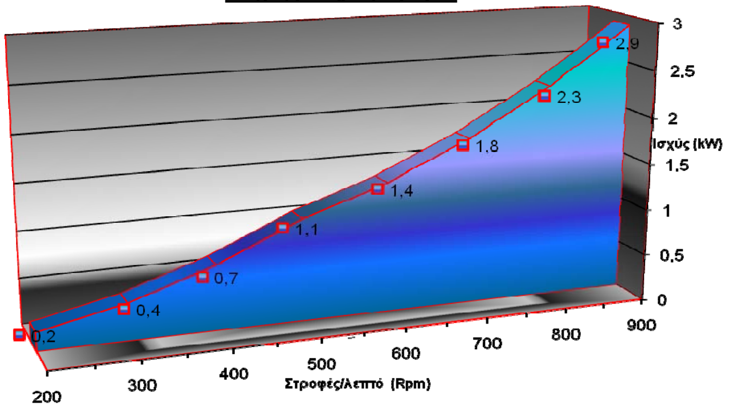
Διάγραμμα Ισχύος-Στροφών
